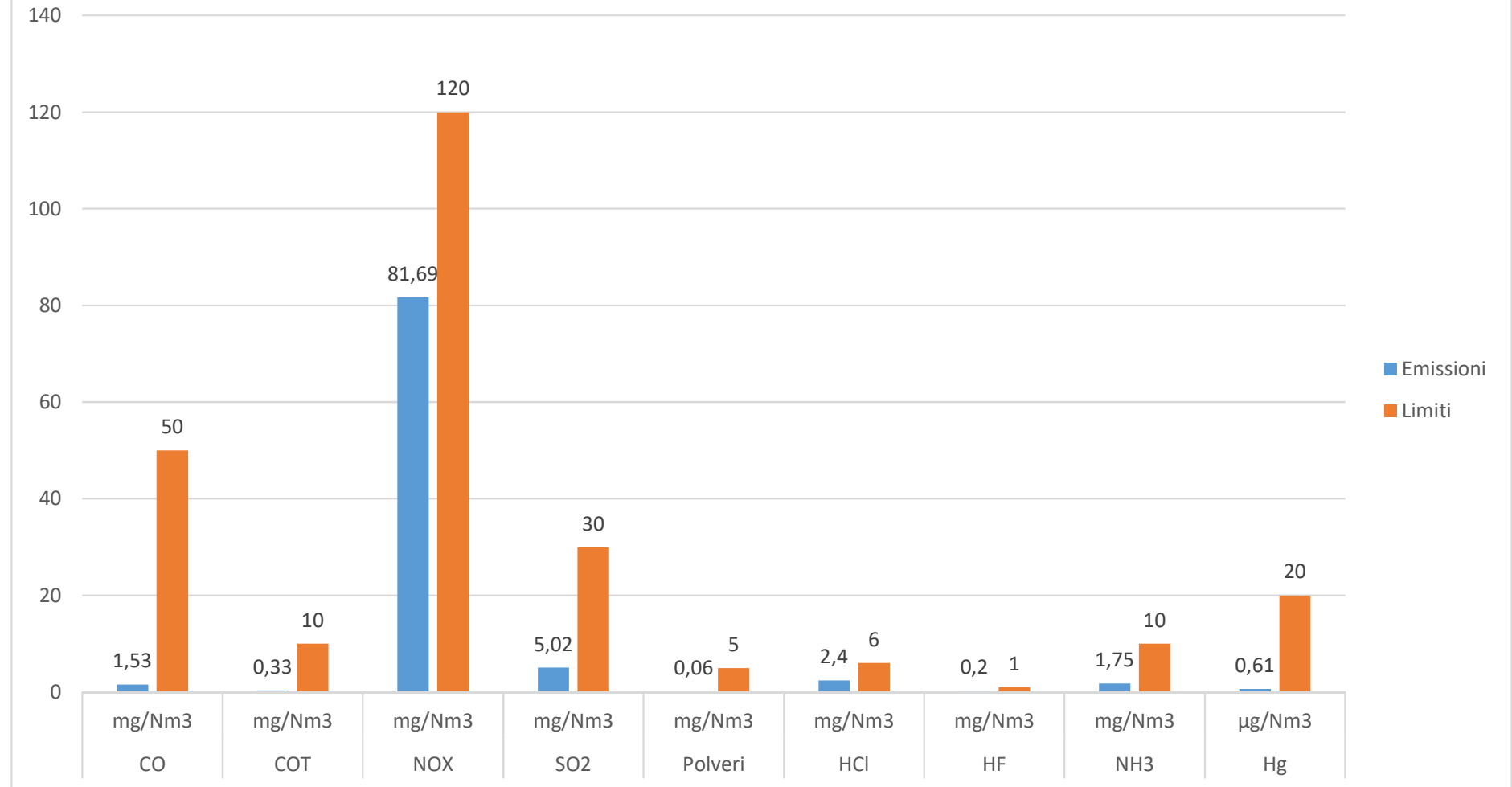
Emissioni CM0 vs Limiti AIA - Novembre 2023
