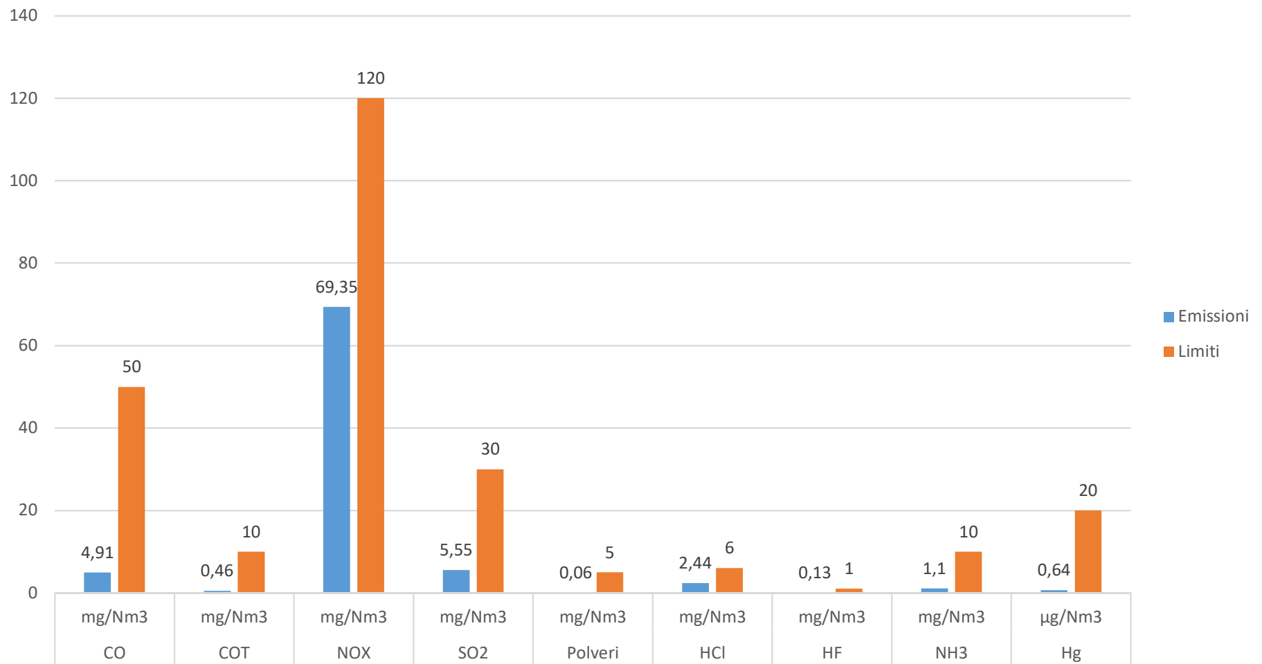
Emissioni CM0 vs Limiti AIA - Settembre 2023
