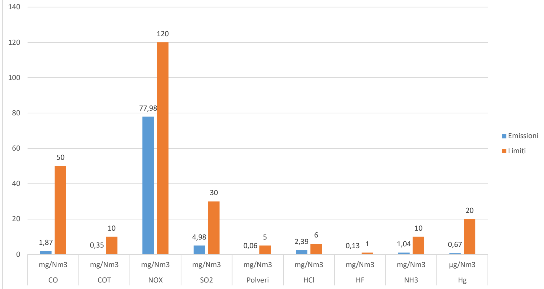
Emissioni CM0 vs Limiti AIA - Agosto 2023
