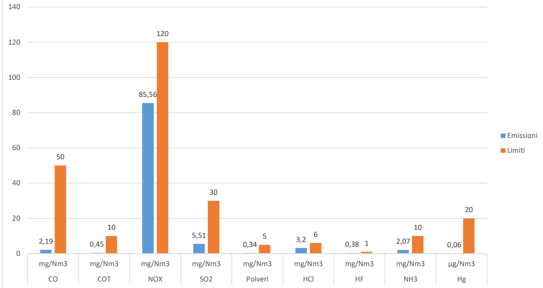
Emissioni CM0 vs Limiti AIA - Maggio 2023
