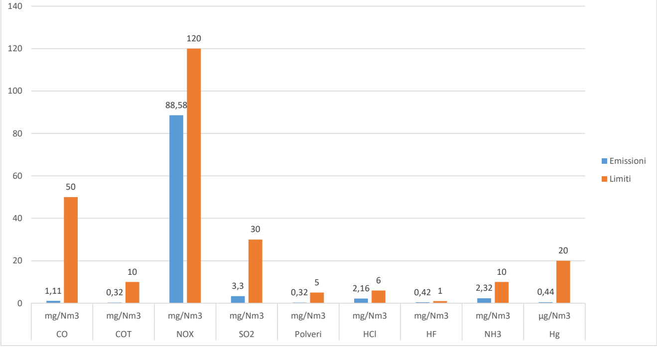
Emissioni CMO vs Limiti AIA - Gennaio 2023
